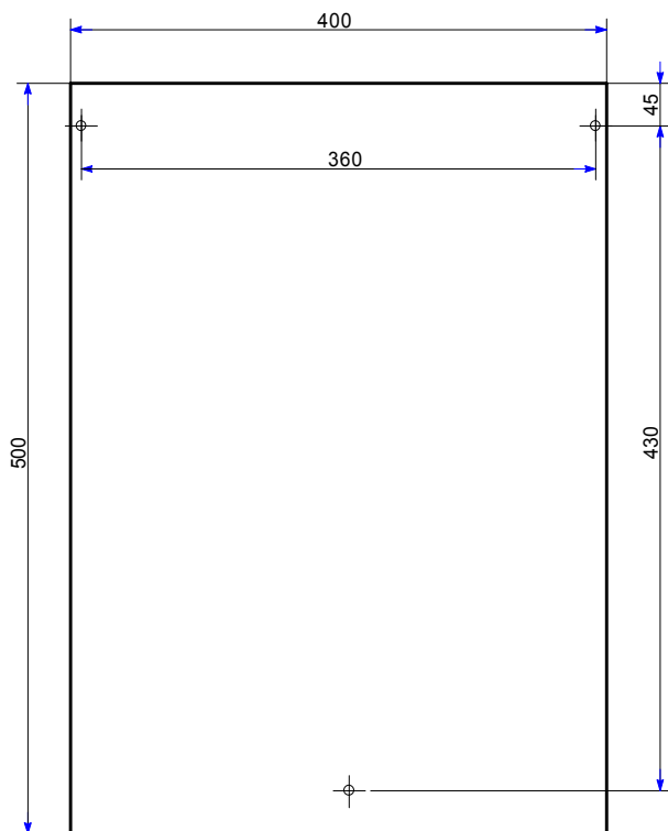
СВТ64.152.000-01(..-08) [1 - 25А]
