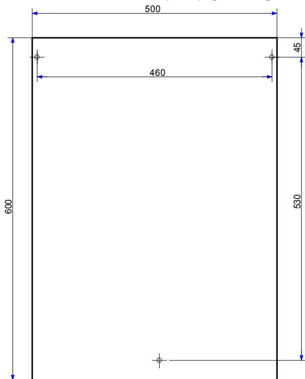
СВТ64.152.000-09(..-13) [32 - 80А]
